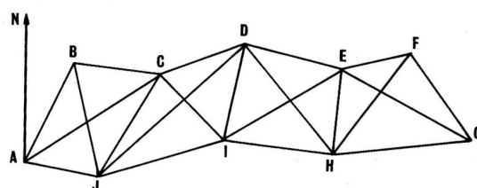
شکل 4-1- تعیین شبکه ژئودزی درجه II
